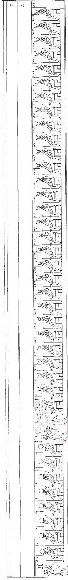
Architrave 3-3'. Série droite, face est
