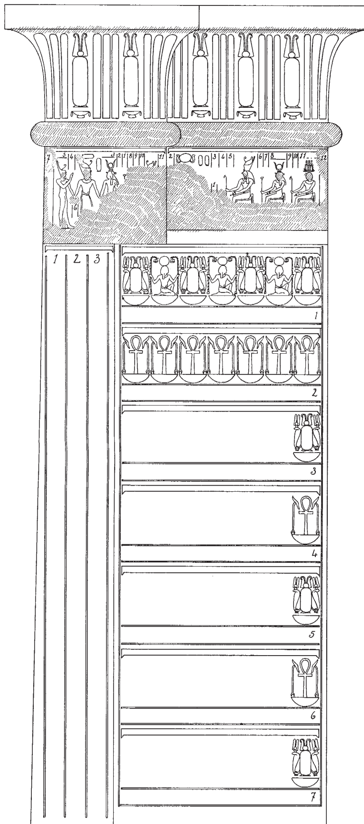
Montant Ouest
