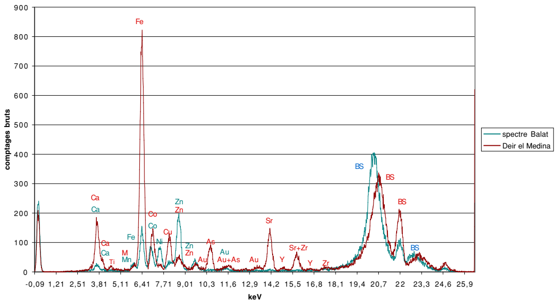
Fig. 74. Spectre comparé de bleu au cobalt.
