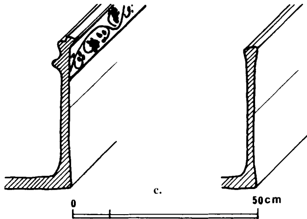
Fig. 9. a-c. Vallée des Reines. Élévations des deux cuves de sarcophages provenant de la tombe n° 13 ; l'une d'elles est décorée d'une frise de rinceaux de vigne et pourvue de poignées intérieures.
