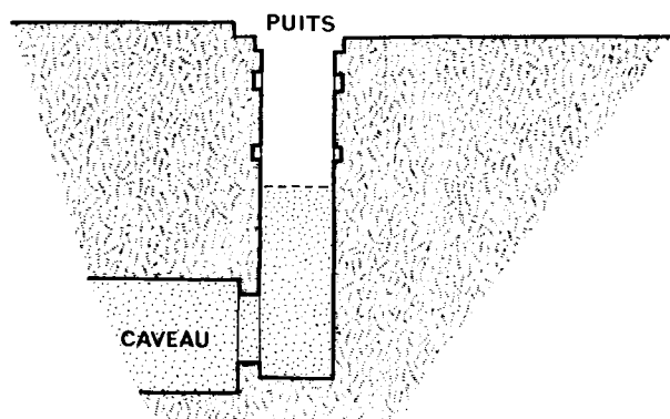
Fig. 1. — Procédé de forage n o 1,
