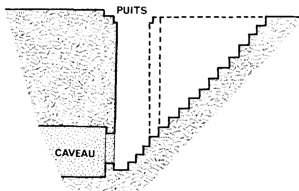
Fig. 2. — Procédé de forage n o 2,
