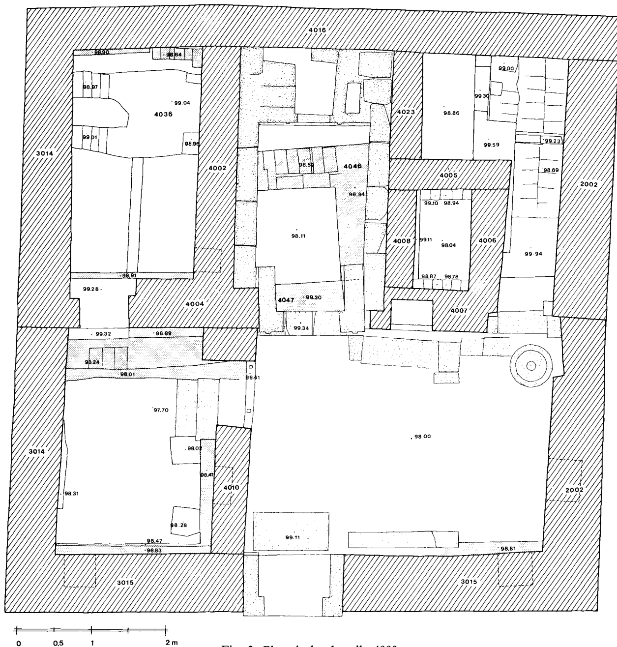
Fig. 3. Plan de la chapelle 4000.
