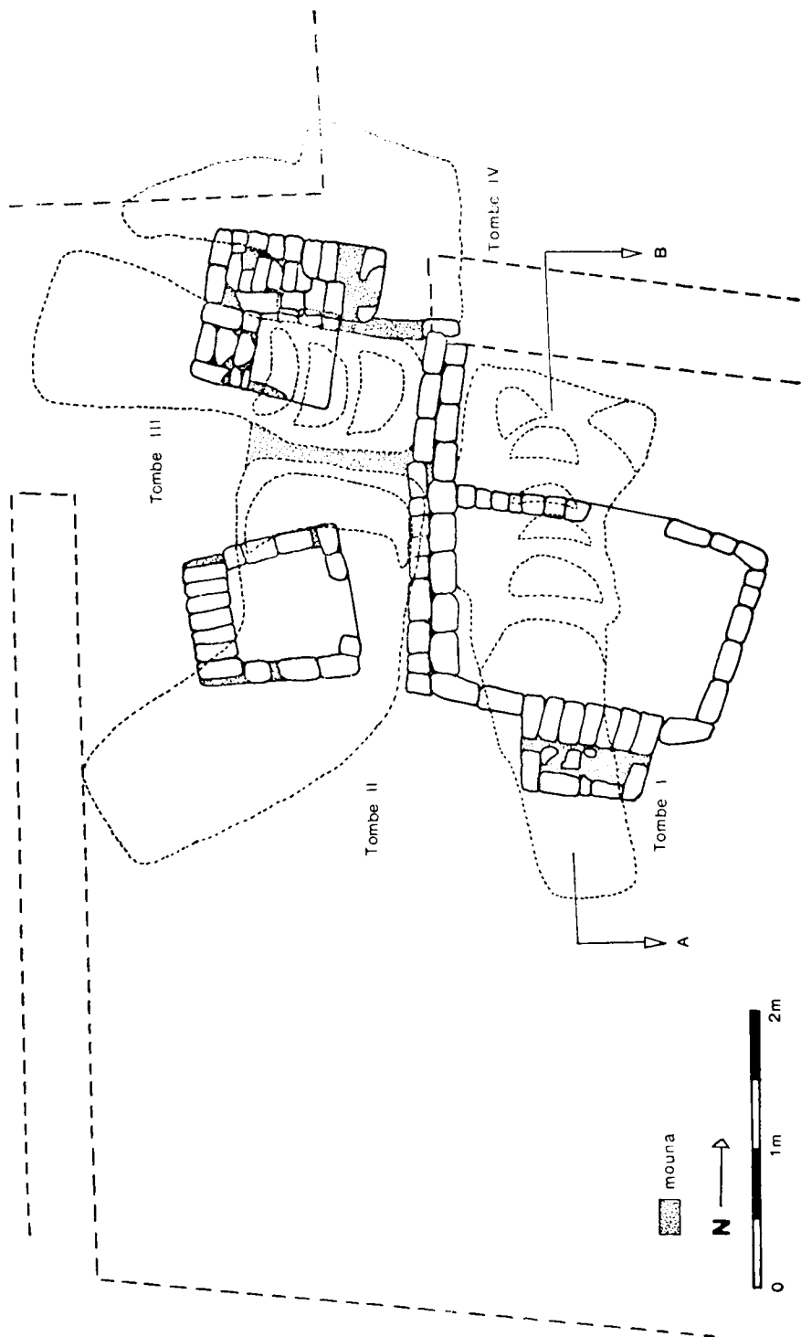
Fig. 1. — Plan d'ensemble des superstructures.
