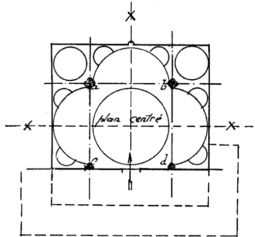
Fig. 15. — Dispositif de coupole, demi-coupoles et trompes de la mosquée de Mihriyah, à Scutari (1547).
