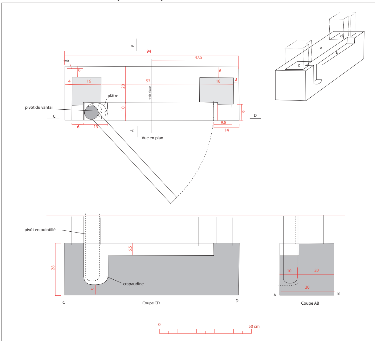
FIG. 19. Détails des plinthes en briques cuites entre les chambres F-G, G-H, H-I, I-J et J-K.
