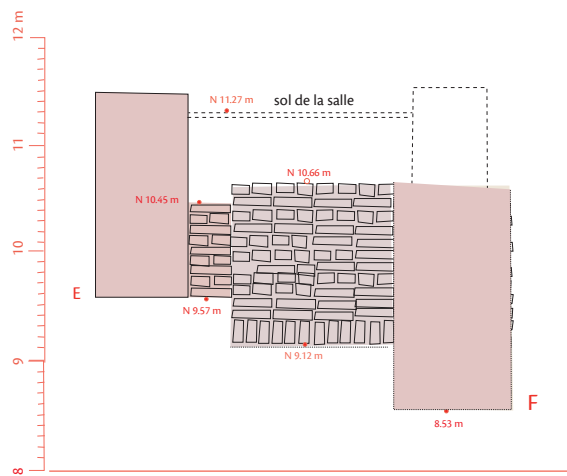
Coupe EF
