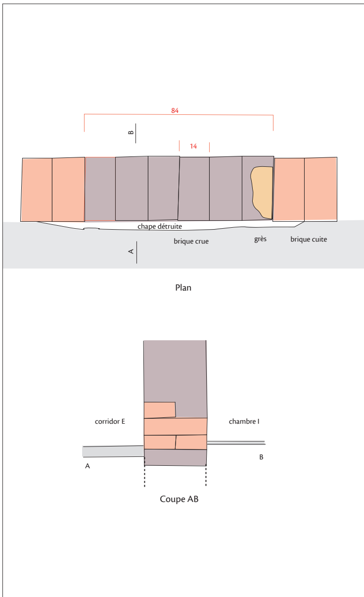
FIG. 23. Plan et coupe du seuil de la porte de la chambre I, détail. Le « sanatorium » de Dendara. Nouvelle interprétation à la lumière d'une étude architecturale © IFAO 2026
