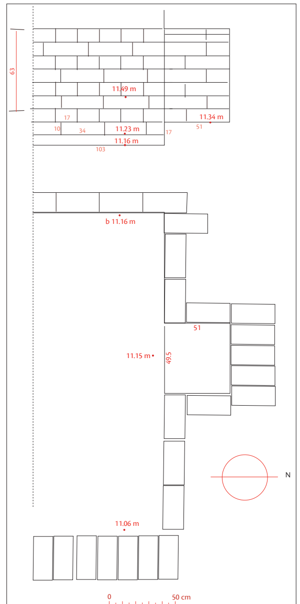
FIG. 24. Plan et élévation du mur ouest de la chambre K. Le « sanatorium » de Dendara. Nouvelle interprétation à la lumière d'une étude architecturale © IFAO 2026 https://www.ifao.egnet.net
