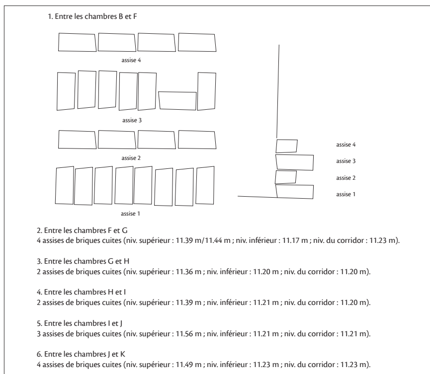
FIG. 19. Détails des pinthes en briques cuites entre les chambres F-G, G-H, H-I, I-J et J-K.
