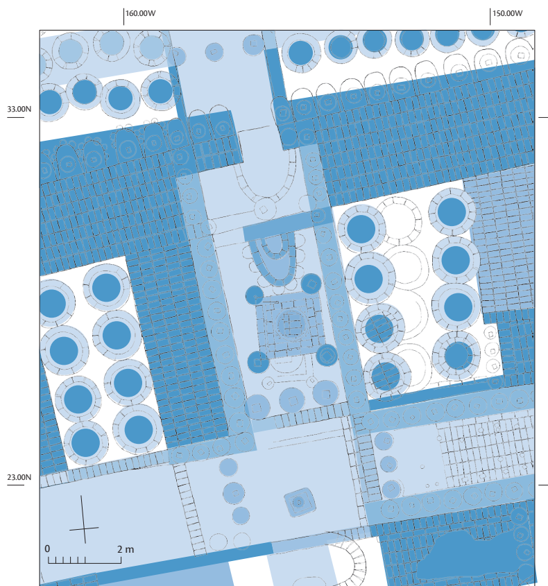
BIFAO 119 (2019), p. 37-49 Fig. 10. Plan des deux chapelles de l'avant-porte nord-ouest. Dessin M. Berti. La porte nord-ouest de la ville antique de Doukki Gel © IFAO 2026
