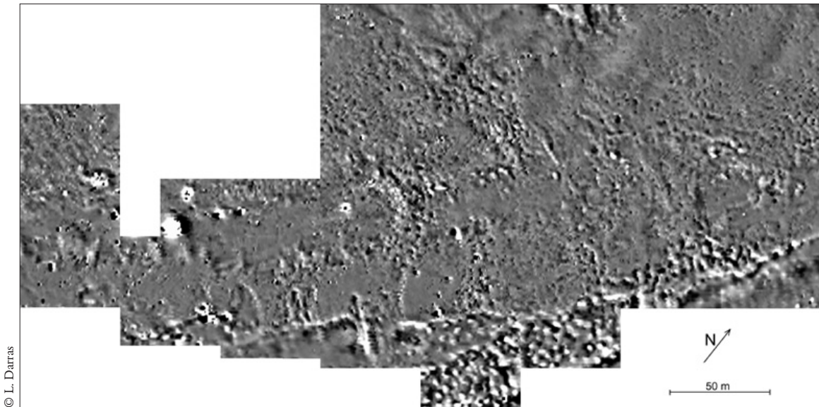
FIG. 12. Carte magnétique brute, -10\text{nT} (blanc)/ +10\text{nT} (noir).
