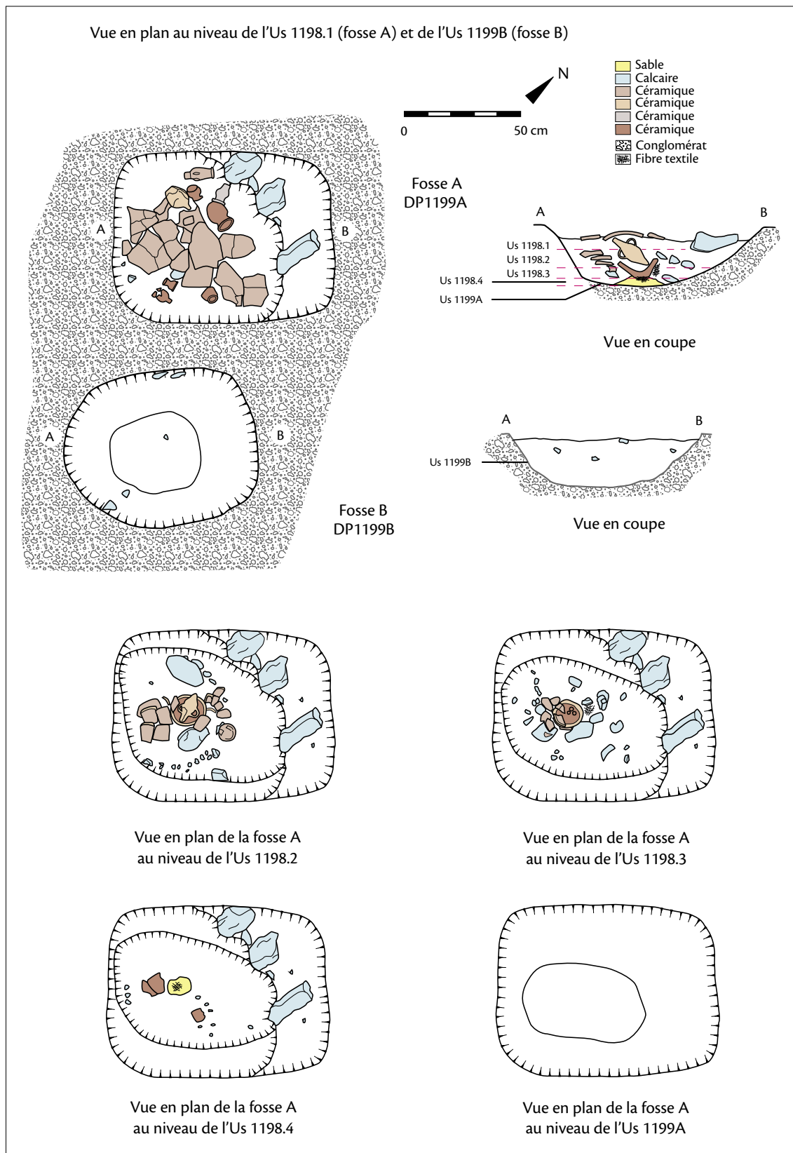
PL. 3. Le dépôt de fondation DP1199 : Plans et coupes (Relevé de terrain/DAO F. Mourot/J.-C. Sztuka 2015).
