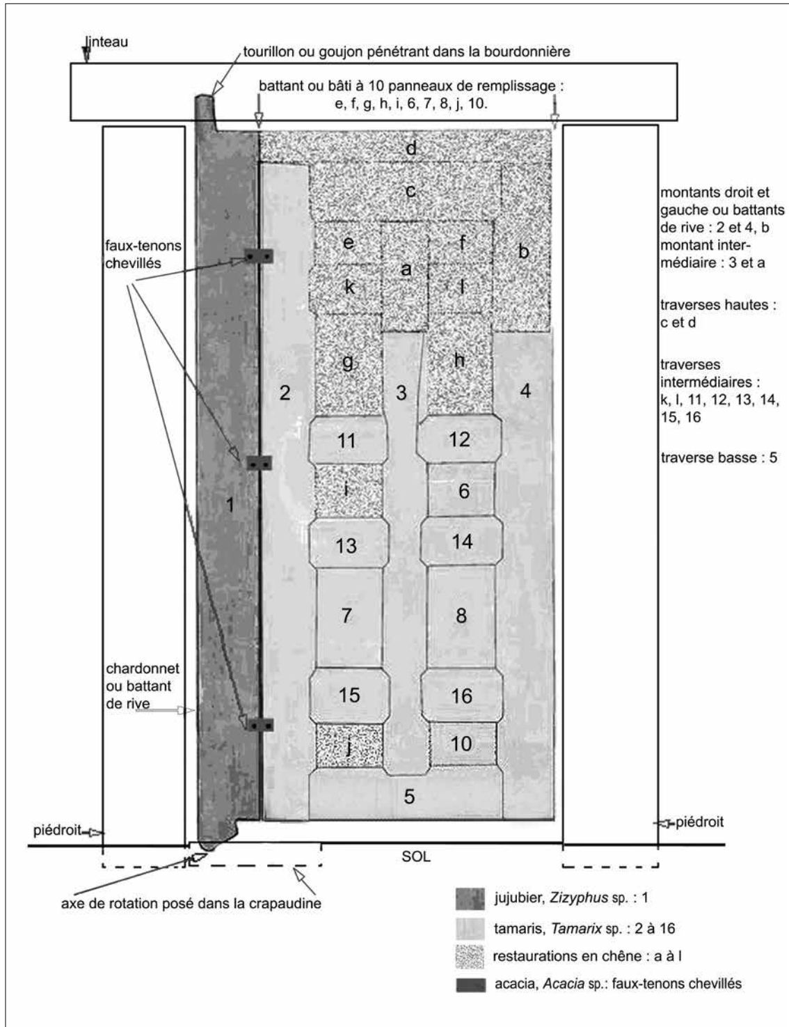
FIG. 3. Désignations et essences sur le schéma du contrepneum.
