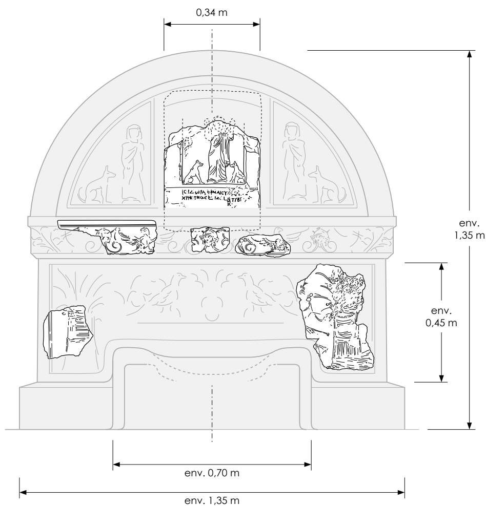
FIG. 6. Tombe d'Isidora, fille d'Hermaios, à superstructure en berceau. Térénouthis - Kom Abou Billou: une ville et sa nécropole. Restitutions d'après photographies et description du Journal Kom Abou Billou d'E. Peterson. © IFAO 2025 BIFAO en ligne https://www.ifao.egnet.net
