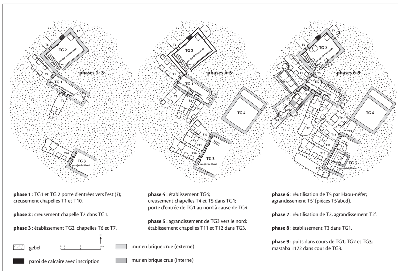
FIG. 12. Détail des différentes phases de construction du complexe de Khnoum-hotep. Travaux de l'Institut français d'archéologie orientale 2008-2009 © IFAO 2026
