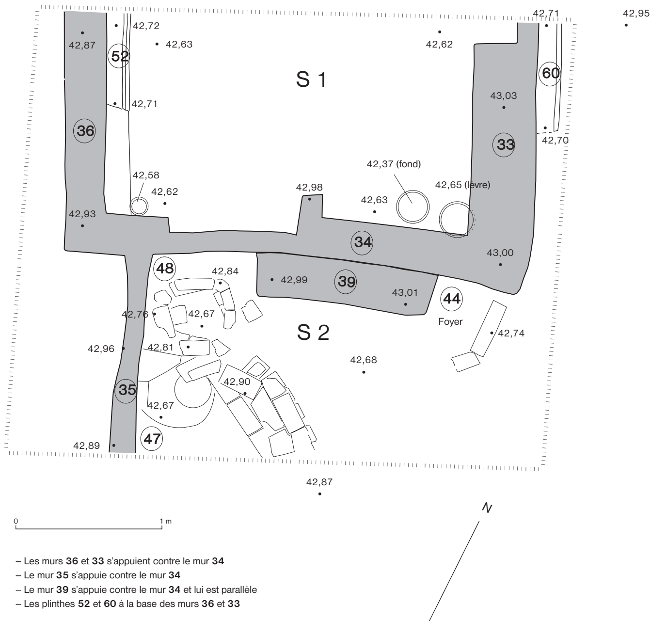
FIG. 17. Plan du sondage 2 par Ramez Boutros.
