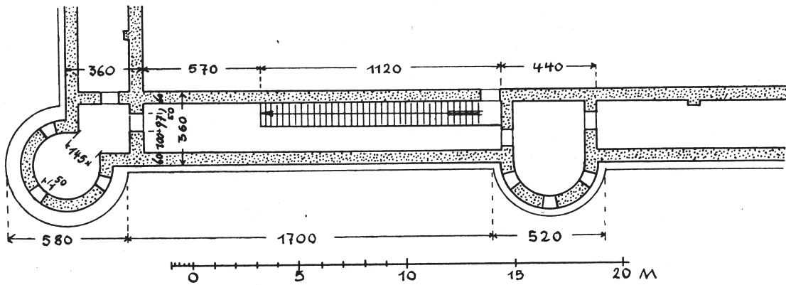
9. Plan d'Ed-Deir, d'après Naumann, MDAIK 8, 1939, pl. 1.
