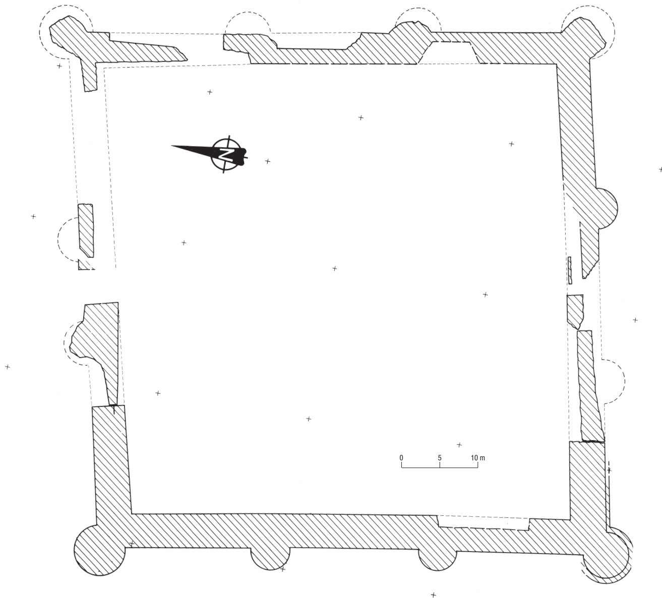
10. Plan général d'Ed-Deir, par Braun, Deleuze, Lecler.
