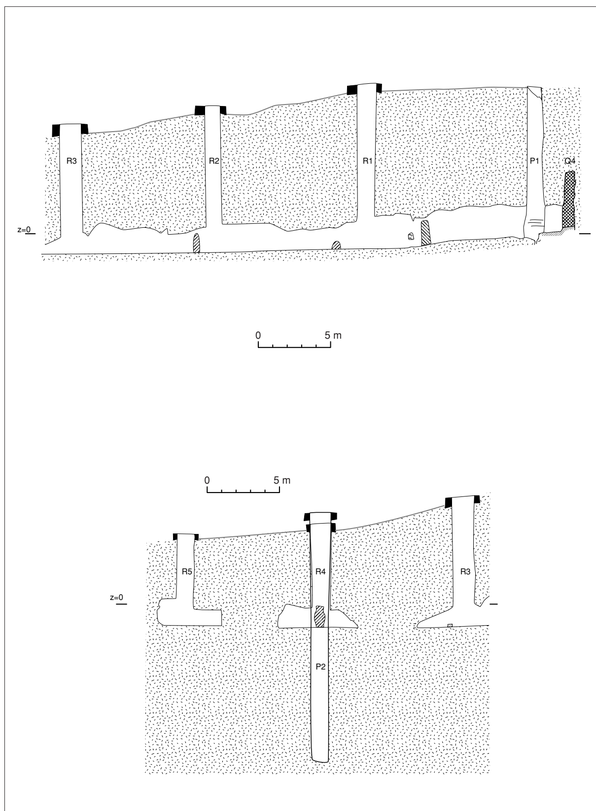
Fig. 42. Coupe longitudinale de la qanat MQ4'.
