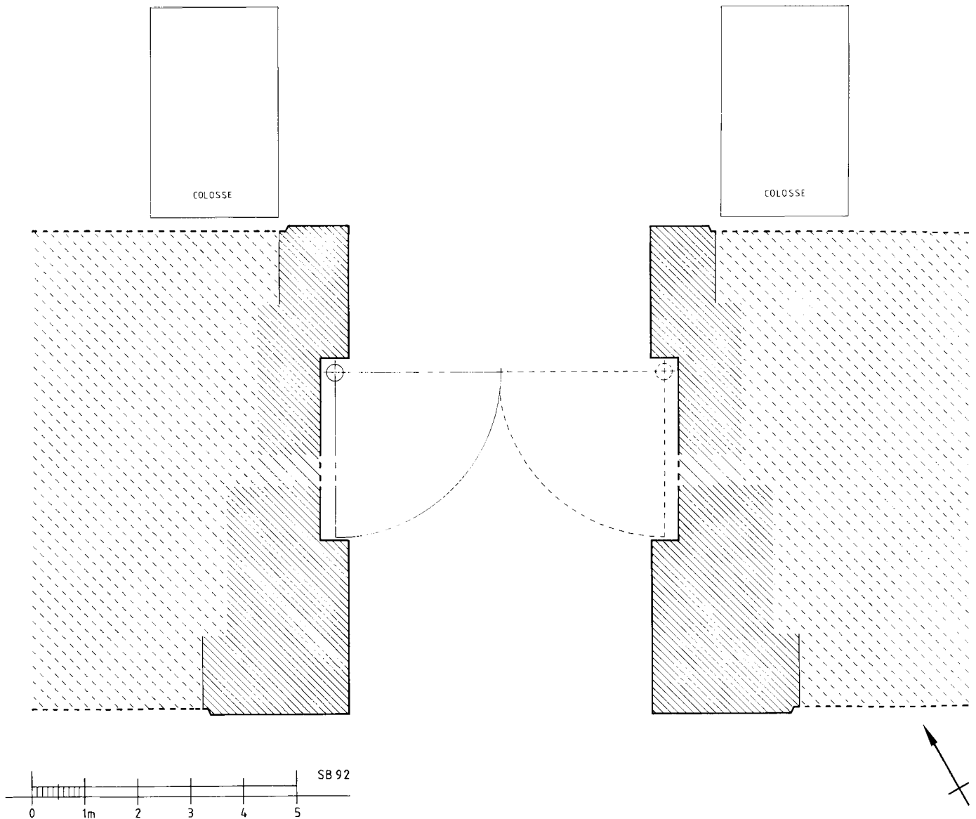
Fig. 5. Restitution du plan de la porte dans un massif de briques.
