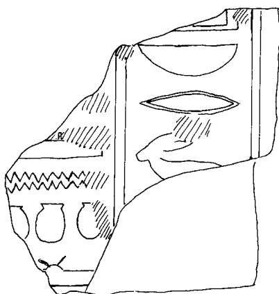
Fragments de colonnes larges non replacés. (Éch. 1/4)
