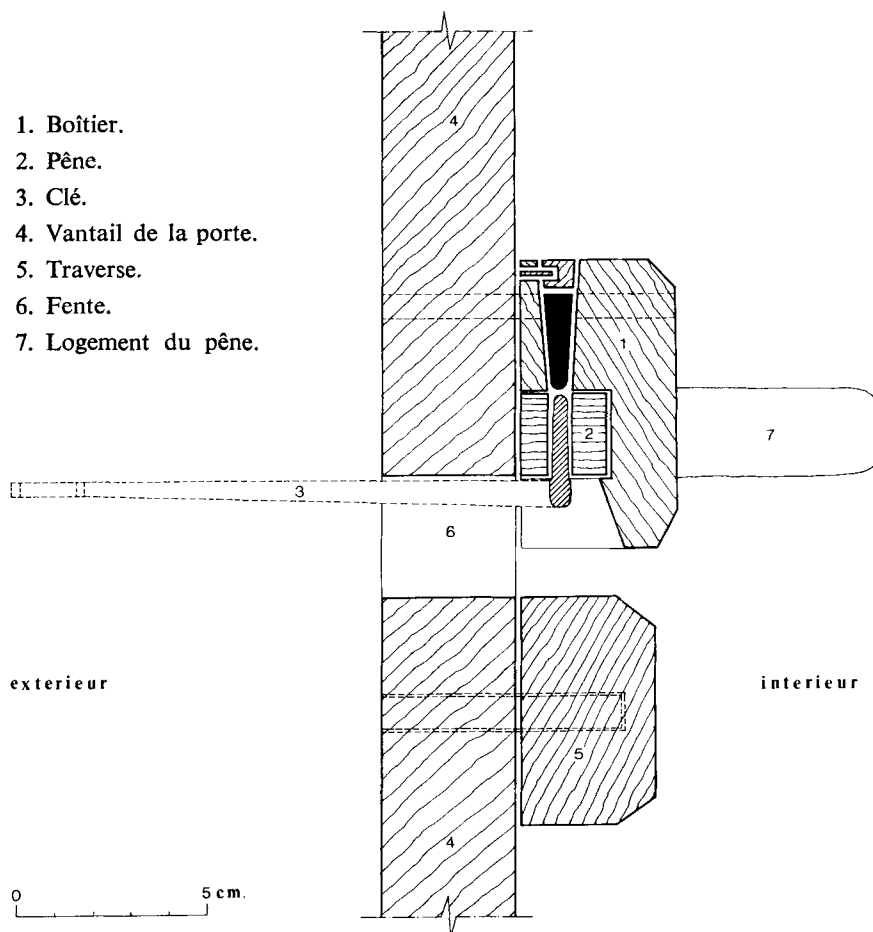
Fig. 16. — Coupe verticale.
