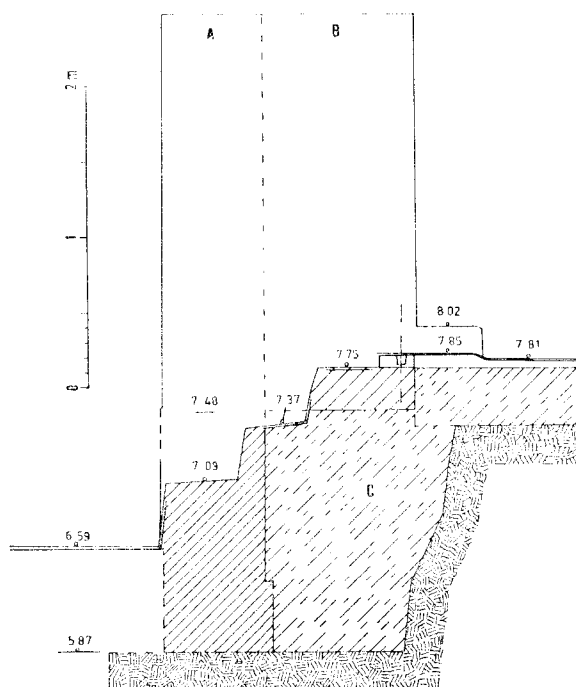
Fig. 9. — Porte de communication entre les deux églises. (A — mur Est de l'église Ouest, B — mur Ouest de l'église Est, C — remplissage).
