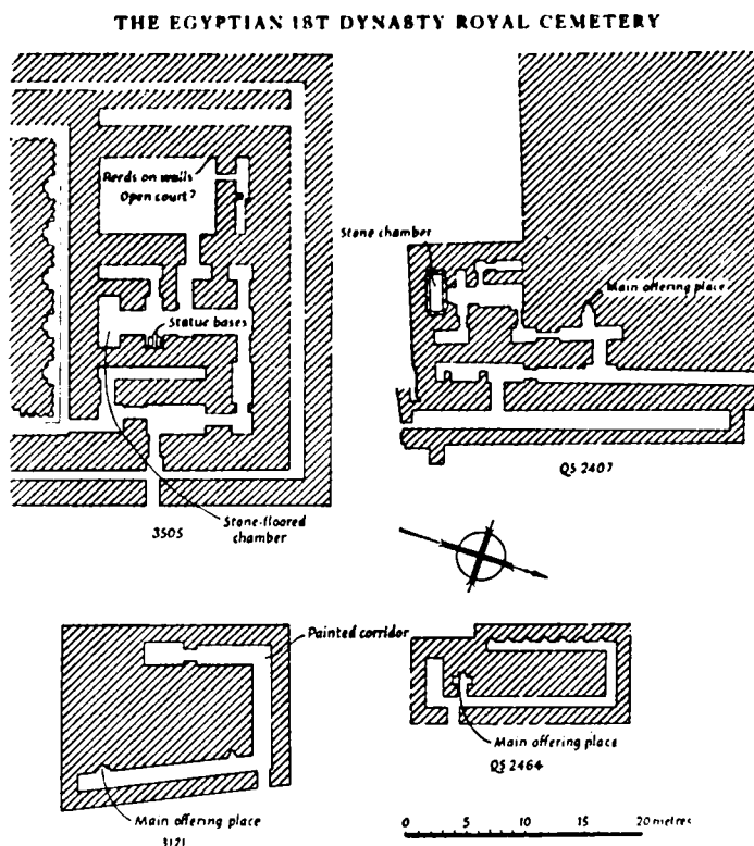
Fig. 5. — Plans comparés du temple funéraire du tombeau de l'Horus Qa-â, n° 3505, du mastaba 3121 (fin I e dynastie) et des mastabas QS. 2407 et 2464 (III e dynastie), d'après Barry J. Kemp.
