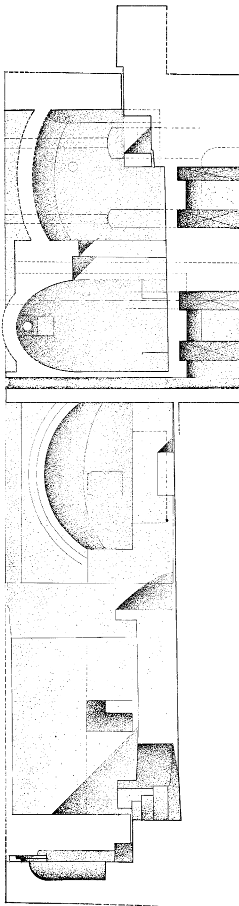
PLAN 7. — Section nord-sud montrant le frigidarium, le laconicum et le caldarium.
