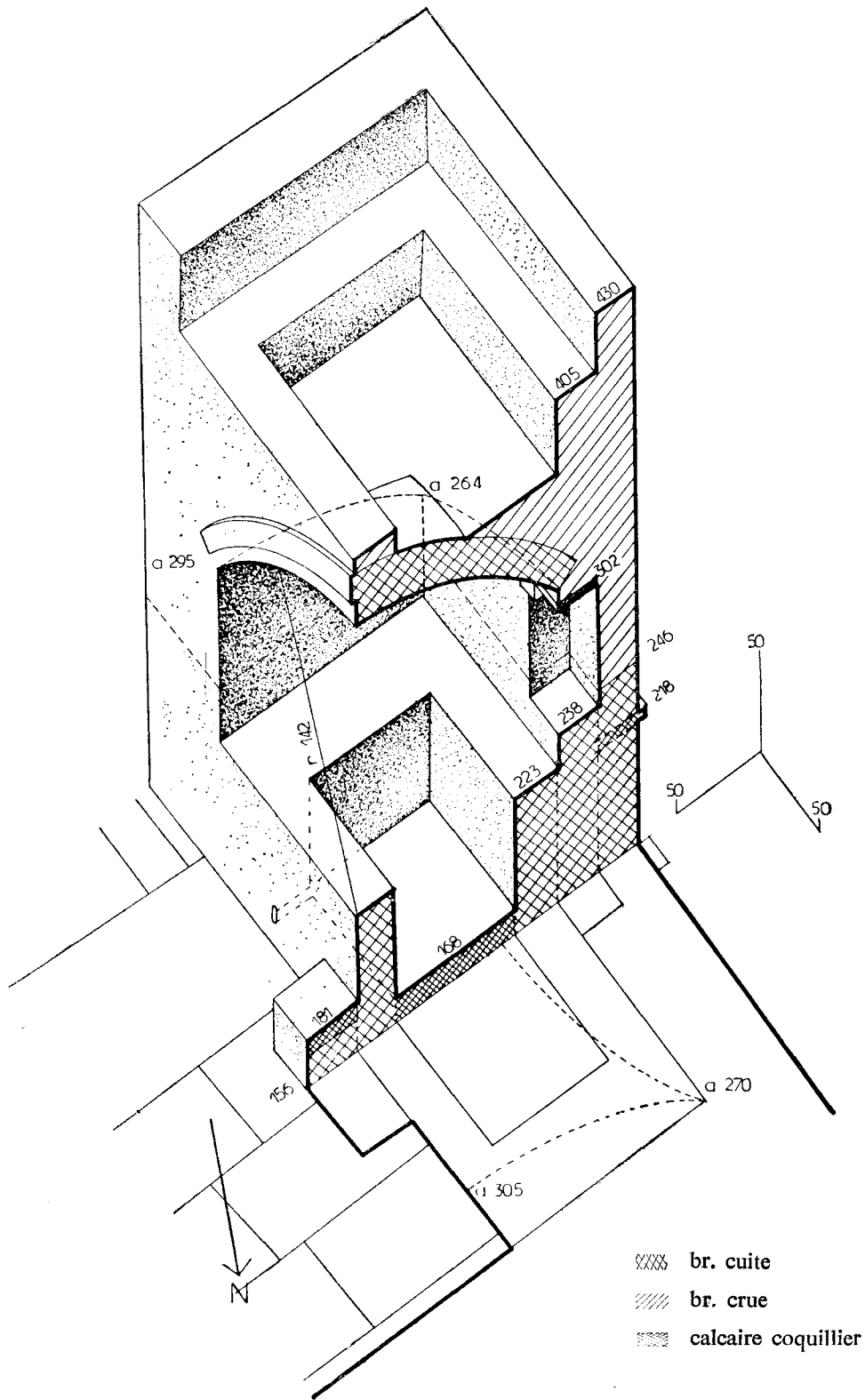
Fig. 2. — Axonométrie, frigidarium.
