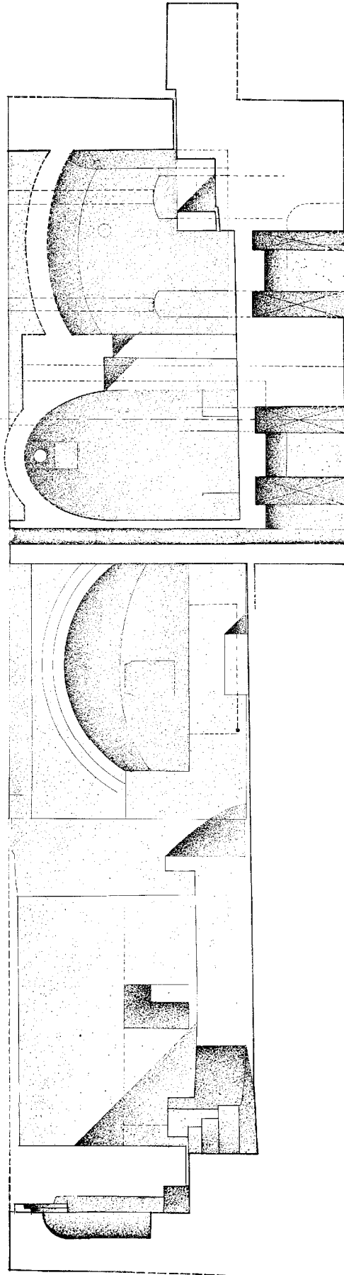
PLAN 6. — Section nord-sud montrant la salle I, le tepidarium et la chaufferie.
