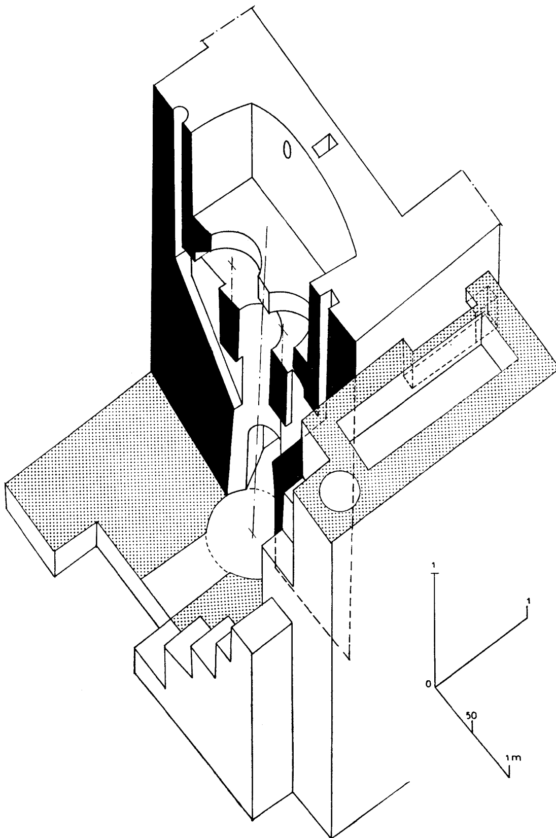
PLAN 14. — Chaufferie, détail.
