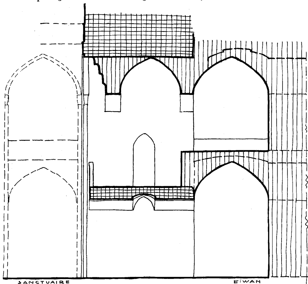
COUPE : C-D - RACCORD DES GALÉRIES DE L'EIWAN AU SANCTUAIRE
