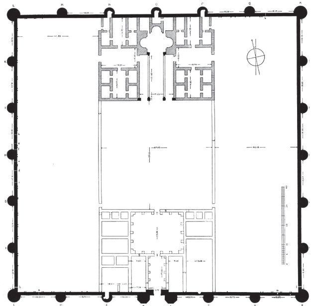
شكل ١٠. مخطط قصر المشتى عن كرزول. قاعة عرش تجمع بين الشكل
