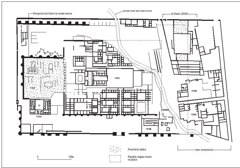
شكل ٢٤. مخطط قصر الجوسق الحاقاني عن نورثدج. Northedge, The Historical Topography of Samarra , p. 142, fig. 59.
