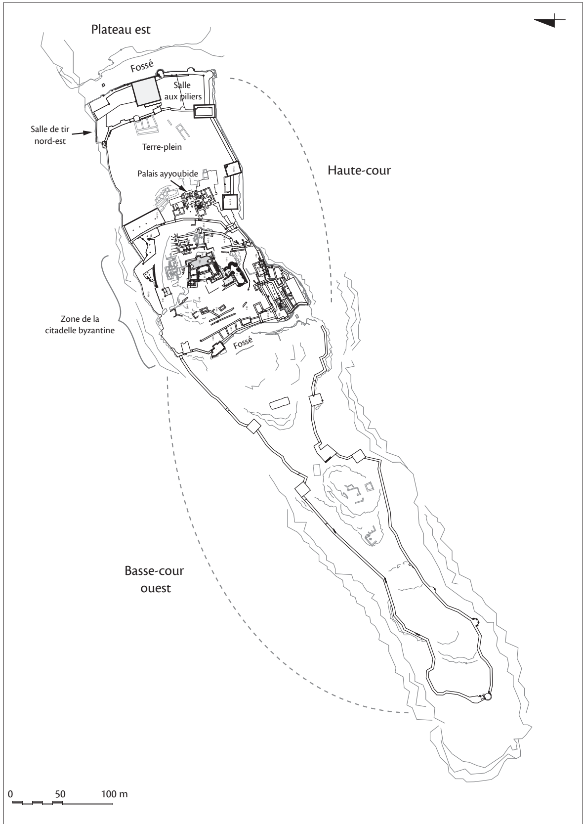
Fig. 2. Plan topographique général du château de Saladin/ Şahyūn / Sa'one (Dessin final : J. Mesqui ; www.castellorient.fr ).
