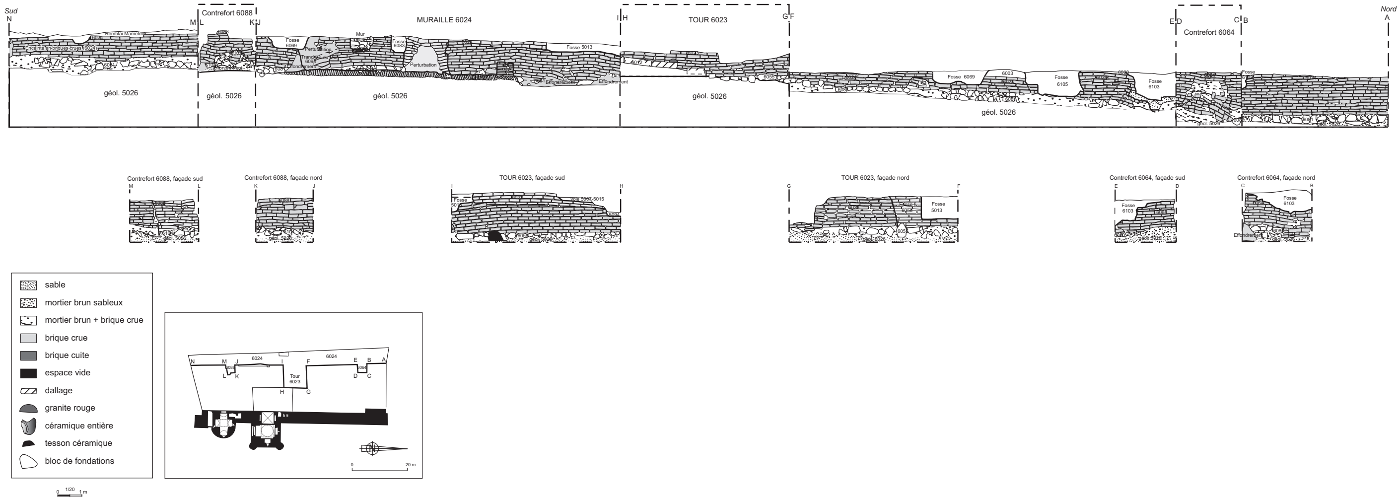
Fig. 30. Élévation de l'enceinte fatimide en briques crues derrière Bāb al-Ġedid.
