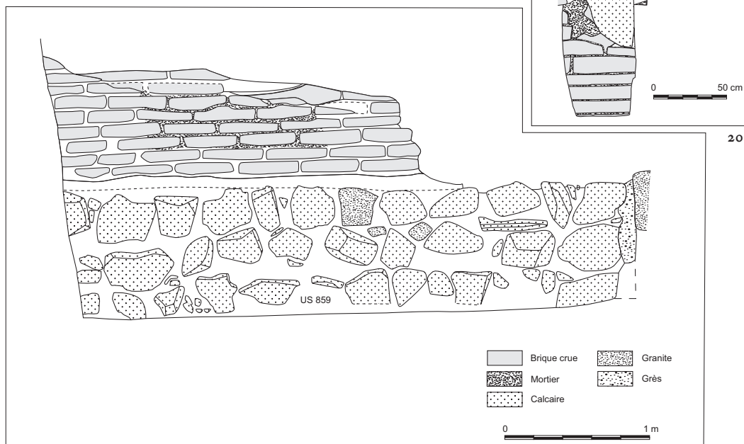
Fig. 19b. Élévation et fondations de la tour au sud de Bâb al-Tawfîq.
