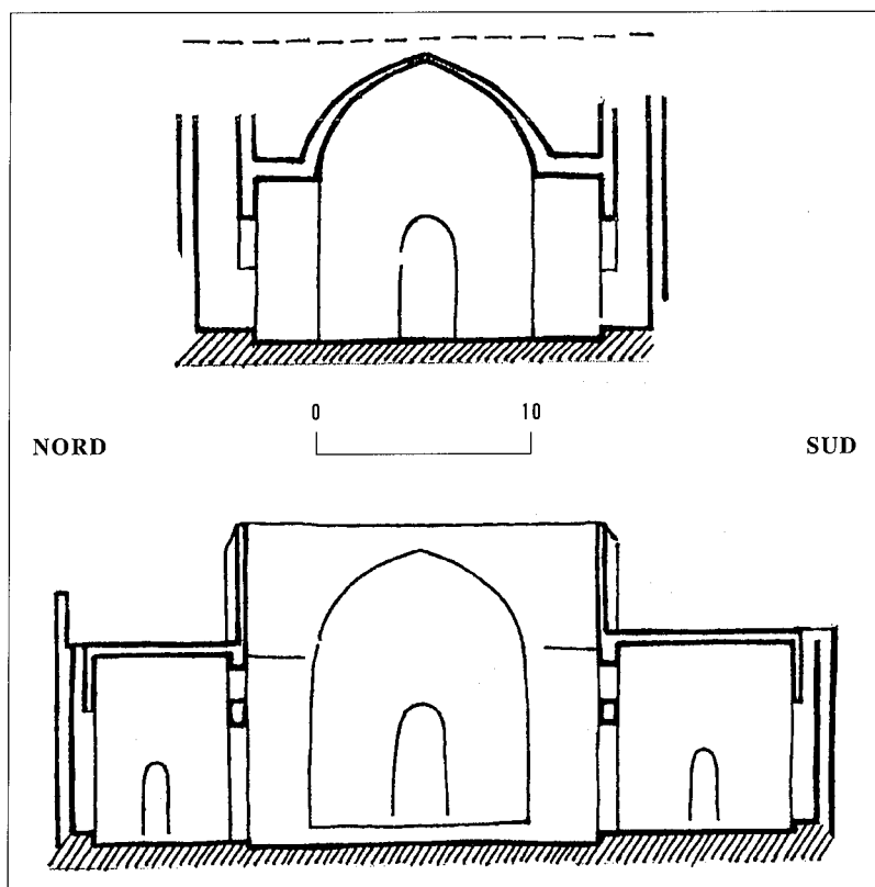
Fig. 9 ▷ Hānqā et mausolée de Baybars al-Ġāṣankir, 1306-1310 ; coupe sur la cour et les maḡlis-s ; coupe sur l'iwān principal et ses deux bādāhang-s.
