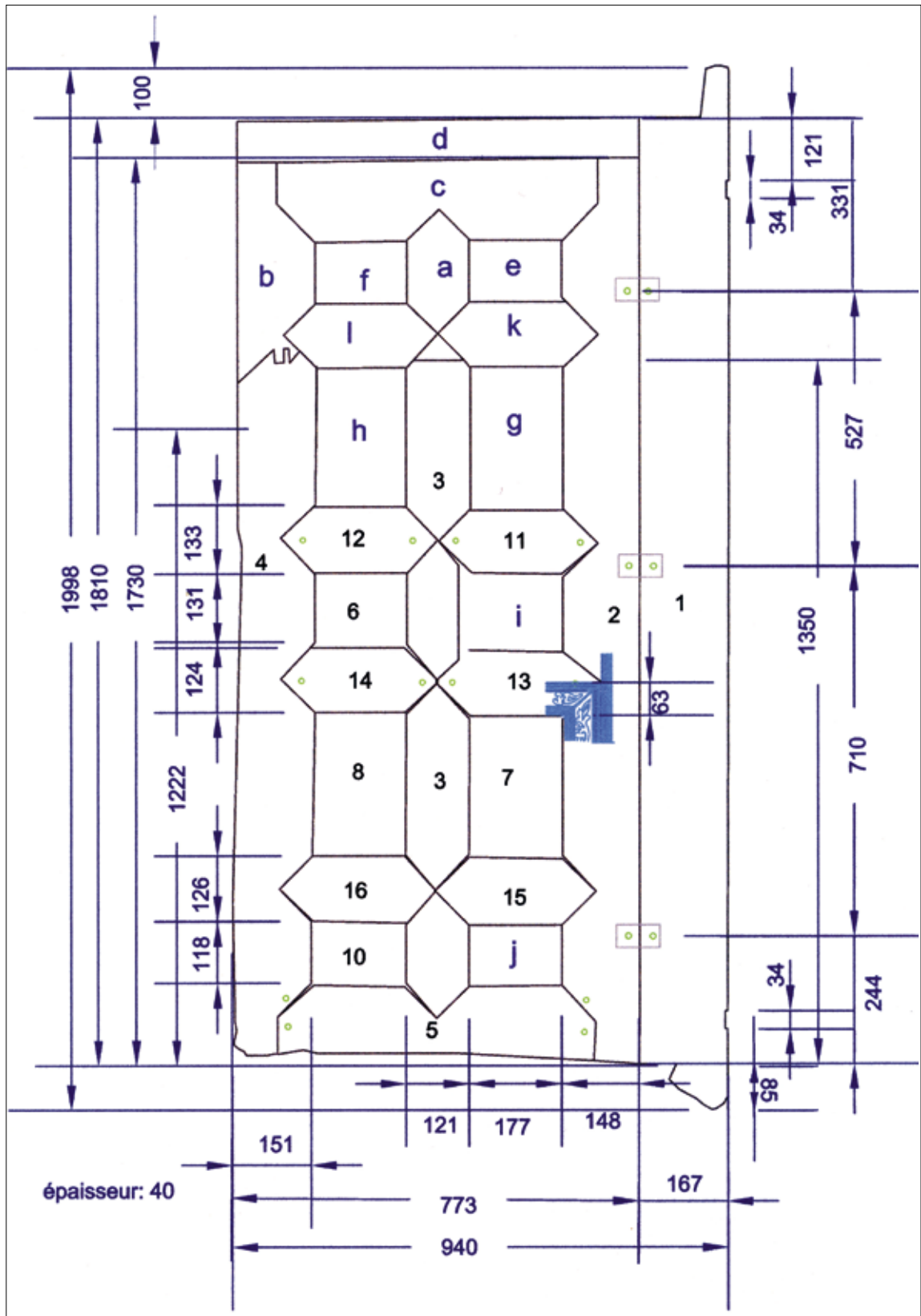
FIG. 4. Relevé coté.
