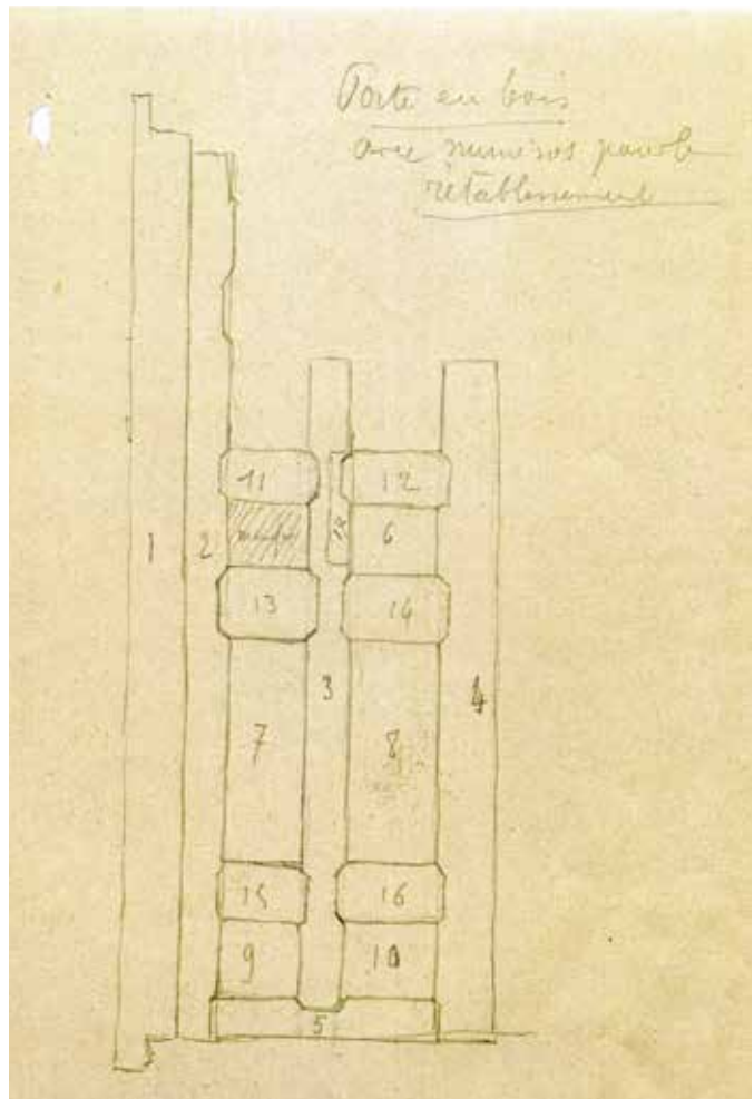
FIG. 2. Croquis pour le remontage (1902). Archives Chassinat, Montpellier.
