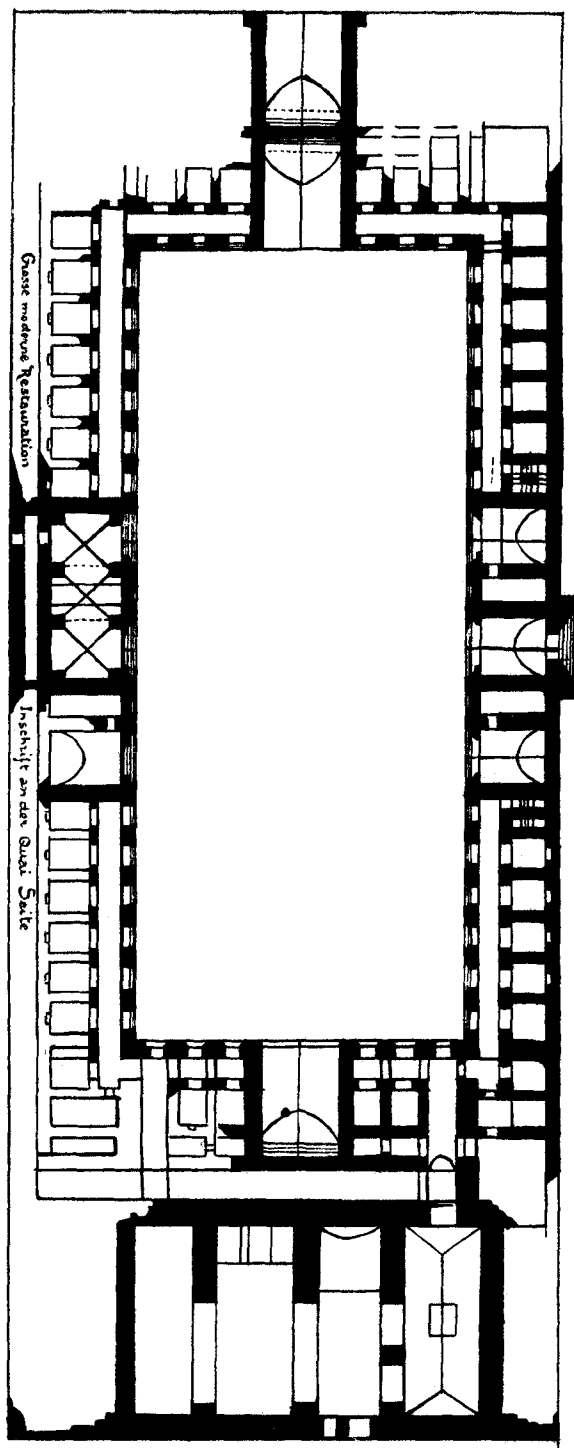
Fig. 9. — BAGHDAD : The Mustansiriya Madrasa. [From SARRE and HERZFELD, Archäologische Reise in Euphrat- und Tigris-Gebiet. ]
